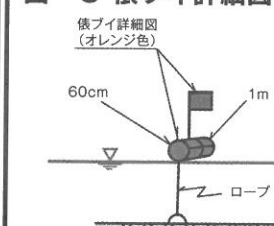
図-5 俵ブイ詳細図
