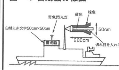
図-4 警戒船の標識
