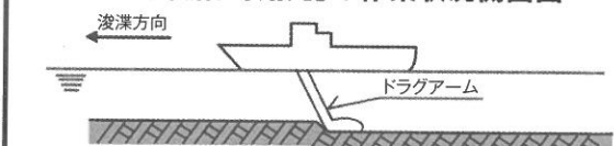
図-7 浚渫船「海翔丸」の作業状況側面図
