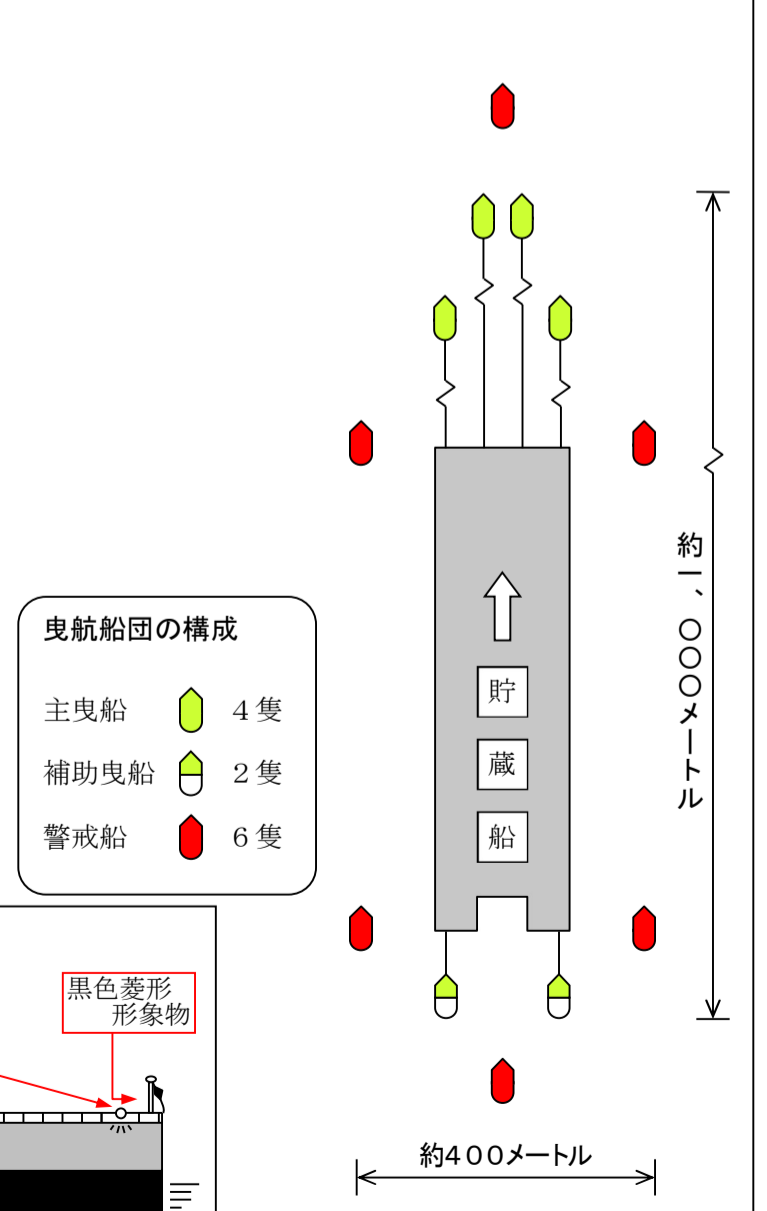
図3 船団構成
