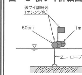
図-5 俵ブイ詳細図
