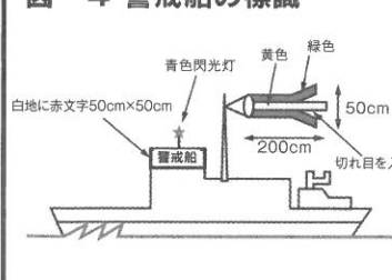
図-4 警戒船の標識
