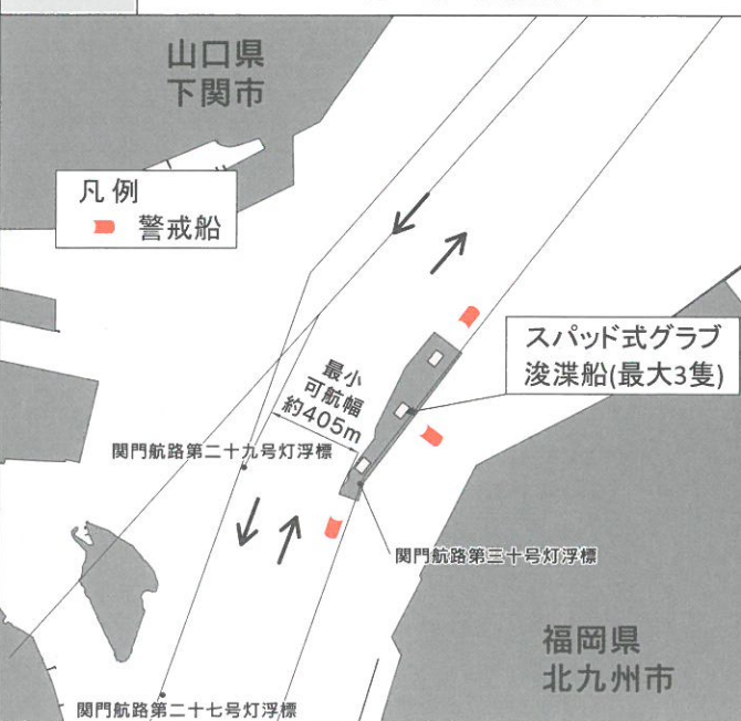
図-3 浚渫船・警戒船配置図【浚渫時の例】 施工時の通航方法
