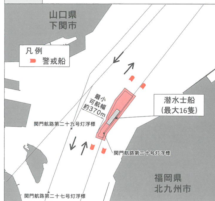
図-2 潜水士船・警戒船配置図【潜水探査時の例】 施工時の通航方法
