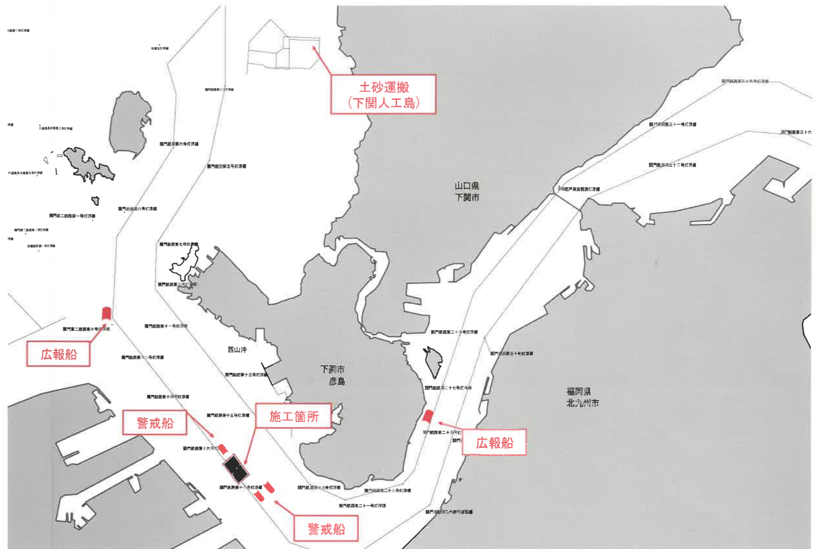
図-1 潜水探査・グラブ浚渫 作業区域図、警戒船・広報船配置図
