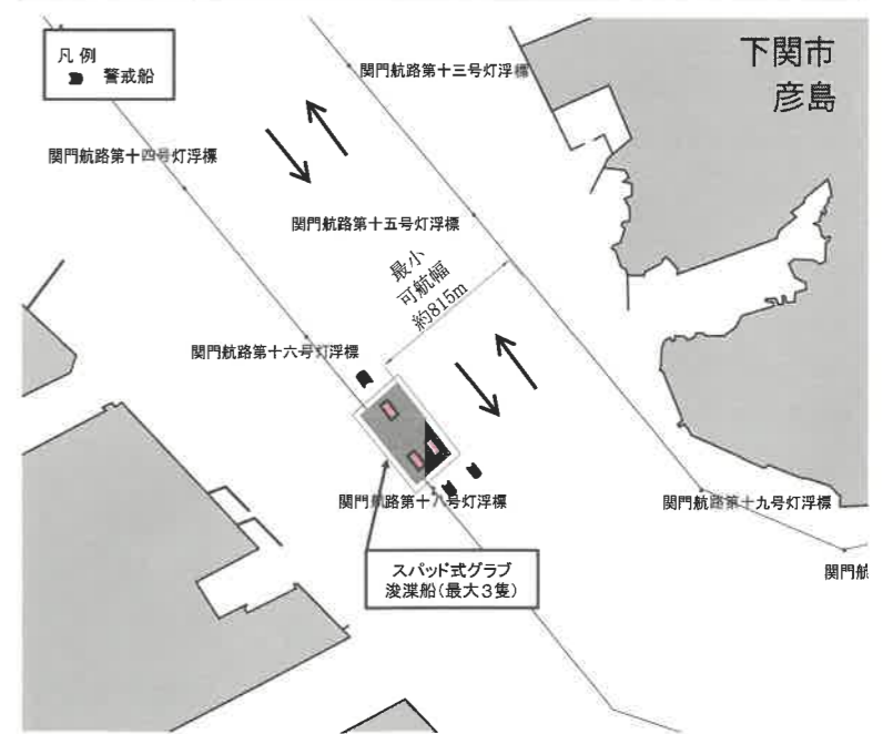
図-3 浚渫船・警戒船配置図【浚渫時の例】 施工時の通航方法【F1・F2・F3工区】
